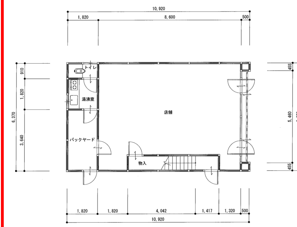
間取り図
